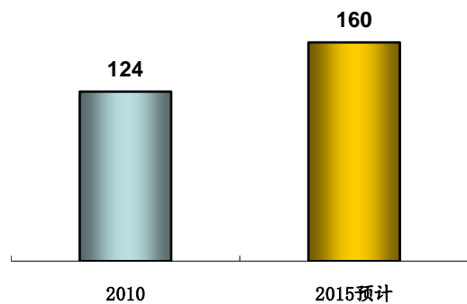
成品油产量
