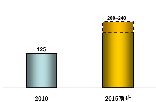
天然气产量
